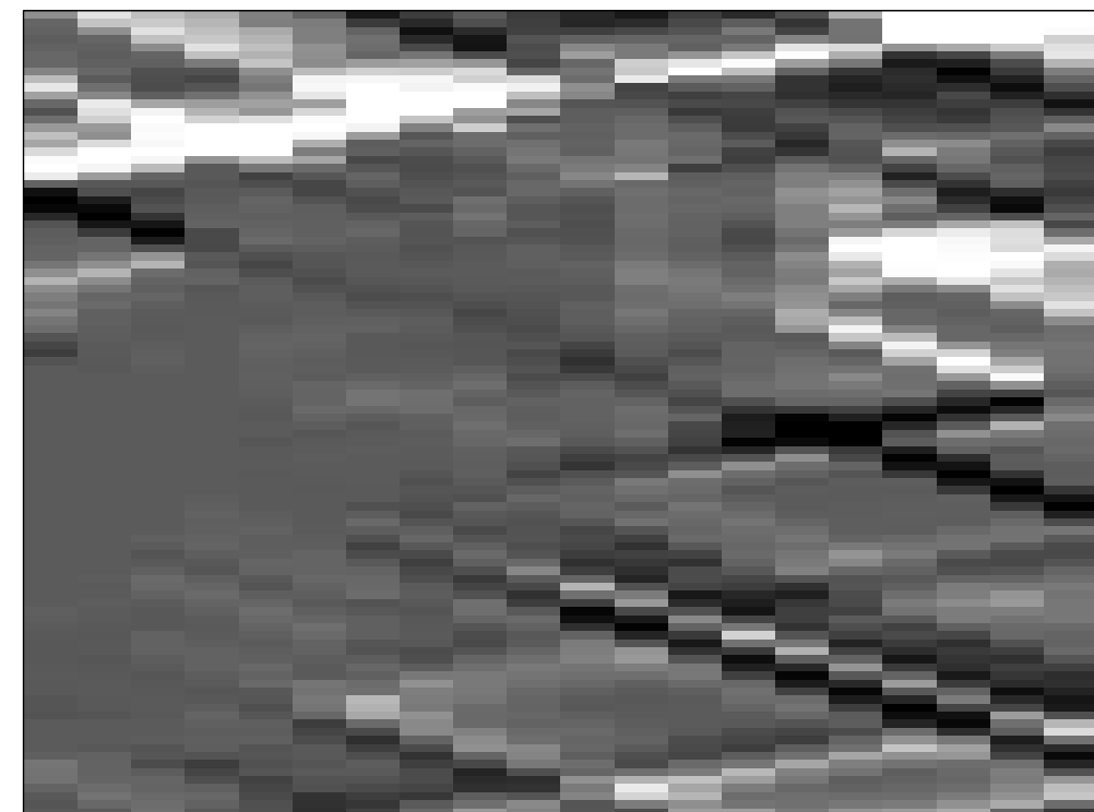
multiscale, iter=1
