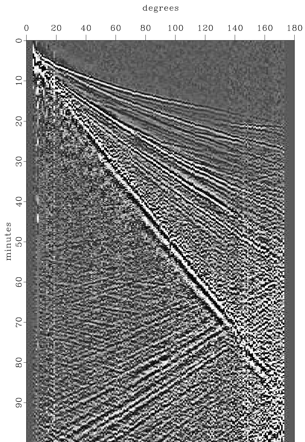
stack (gpow=0.5)
