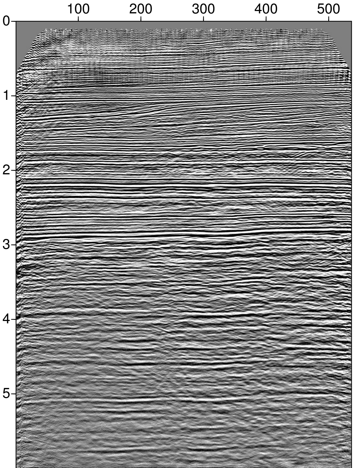
brutestack
