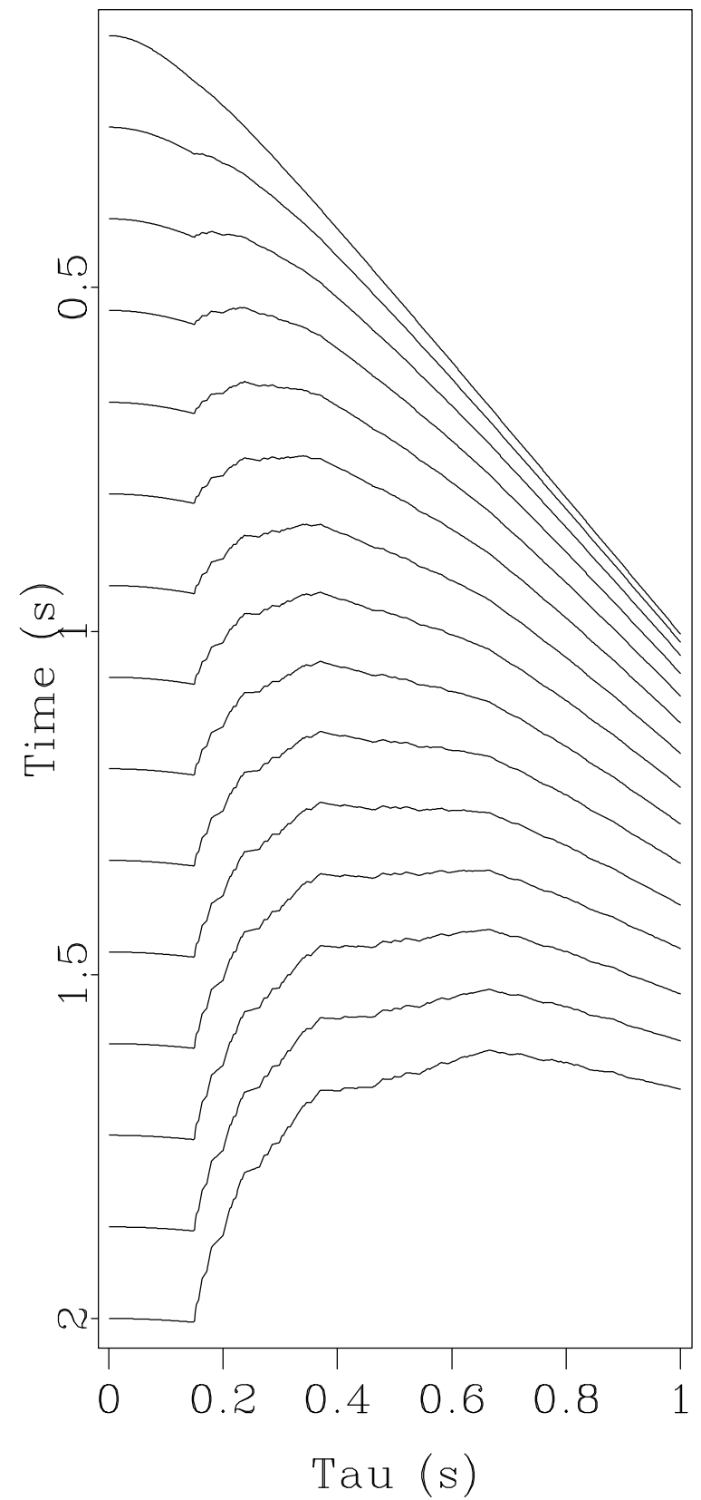
t(\tau)
